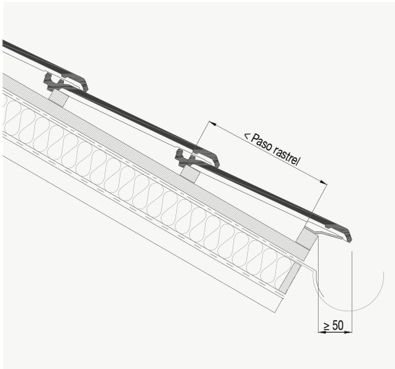
ENCUENTRO HORIZONTAL
