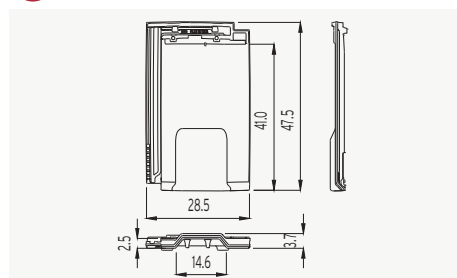
24 Ventilación FLAT-10
