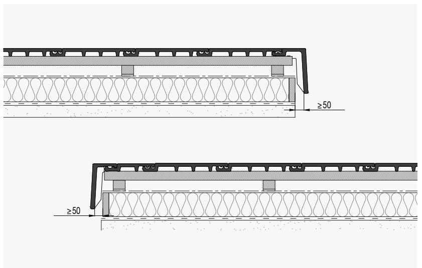
LATERALES
