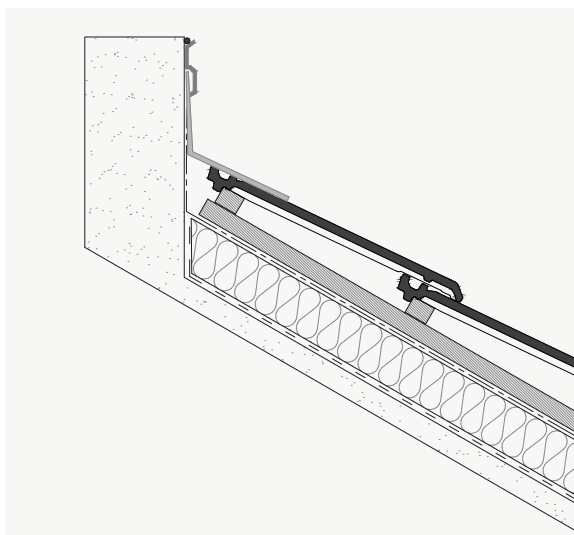
ENCUENTRO SUPERIOR
