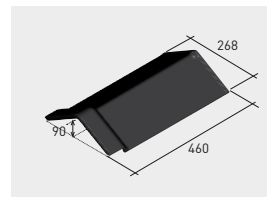
Q110*K | Cumbreira ática encaje alzado klinker
