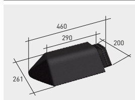
Q109*K | Remate cumbreira ática 120° klinker
