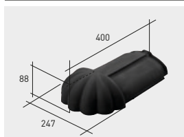
Q03*K | Remate cumbreira klinker
