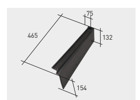
Q116*K | Remate lateral derecho Innova/Vienna klinker
