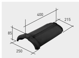
Q01*K | Cumbreira klinker
