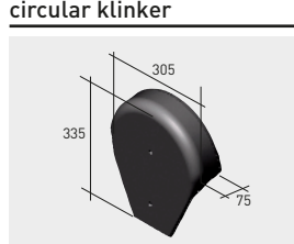
Q83*K | Tapón cumbreira circular klinker
