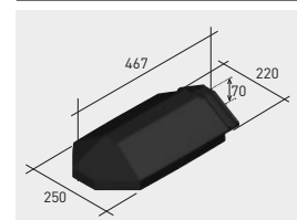
Q122*K | Remate cumbreira angular klinker
