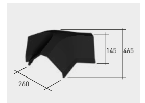
Q146*K | Cumbre pirámide a 3 aguas klinker
