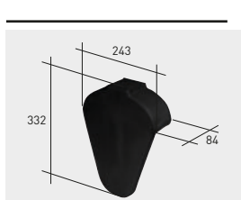
Q05*K | Tapón klinker
