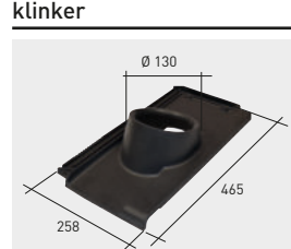
Q118*K | Teja soporte chimenea Innova/Vienna klinker
