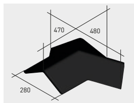
Q111*K | Cumbre ática 120° a 3 aguas klinker
