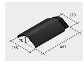
Q120*K | Cumbreira angular klinker
