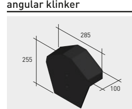
Q124*K | Tapón cumbreira angular klinker
