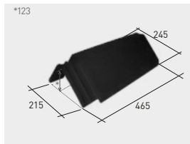
Q145*K | Cumbre 45° klinker
