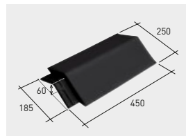
Q90*K | Cumbreira ática 120° klinker
