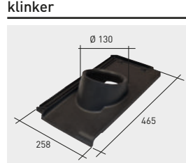
Q118*K | Teja soporte chimenea Innova/Vienna klinker
