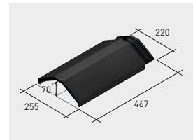
Q120*K | Cumbre angular klinker
