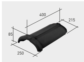
Q01*K | Cumbre klinker
