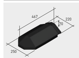
Q122*K | Remate cumbre angular klinker
