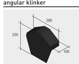
Q124*K | Tapón cumbre angular klinker
