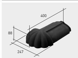
Q03*K | Remate cumbre klinker
