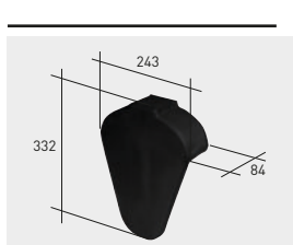
Q05*K | Tapón klinker
