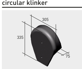
Q83*K | Tapón cumbre circular klinker
