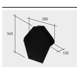
Q147*K | Tapón 45° klinker
